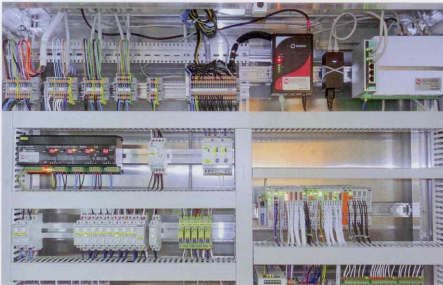
Blick in den Schaltschrank von hbTec AG (sacralis) mit den Universal-Dimmern UDK-04-10 von se Lightmanagement AG. Der UDK-04-10 erlaubt, in Kombination mit den LCC- Leuchtmitteln, das Kirchenschiff von 0 bis 100% stufenlos, flackerfrei und somit zuverlässig zu dimmen.
